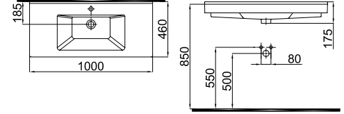
0201-5005 Merkür Lavabo / Merkur Washbasin (46x100)
