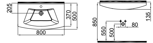
2801-0805 Vega Lavabo / Vega Washbasin (50x80)
