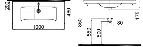
0201-1005 Hera Lavabo / Hera Washbasin (46x100)
