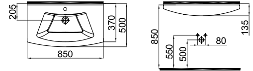
2801-0855 Vega Lavabo / Vega Washbasin (50x85)
