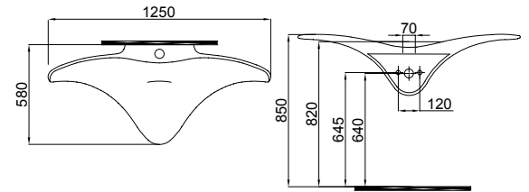
6101-1255 Mialuce Manta Monoblok Lavabo / Mialuce Manta Monoblock Washbasin (58x125)
