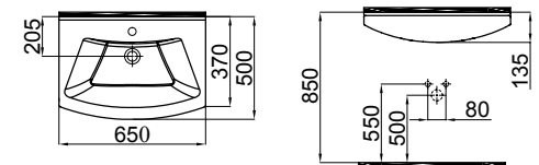
2801-0655 Vega Lavabo / Vega Washbasin (50x65)
