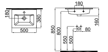
0201-4505 Merkür Lavabo / Merkur Washbasin (38x50)
