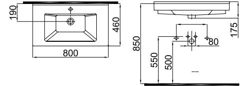
0201-3805 Merkür Lavabo / Merkur Washbasin (46x80)
