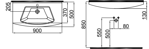
2801-0905 Vega Lavabo / Vega Washbasin (50x90)
