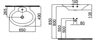
2901-0505 Rena Tezgah Üstü Lavabo / Rena Countertop Washbasin (49x65)
