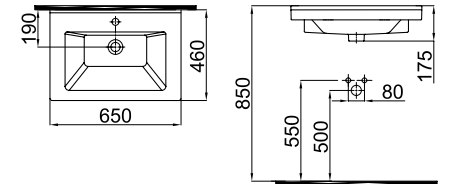
0201-5655 Merkür Lavabo / Merkur Washbasin (46x65)
